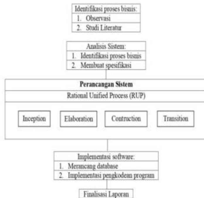
Gambar 1. Kerangka Pemikiran
